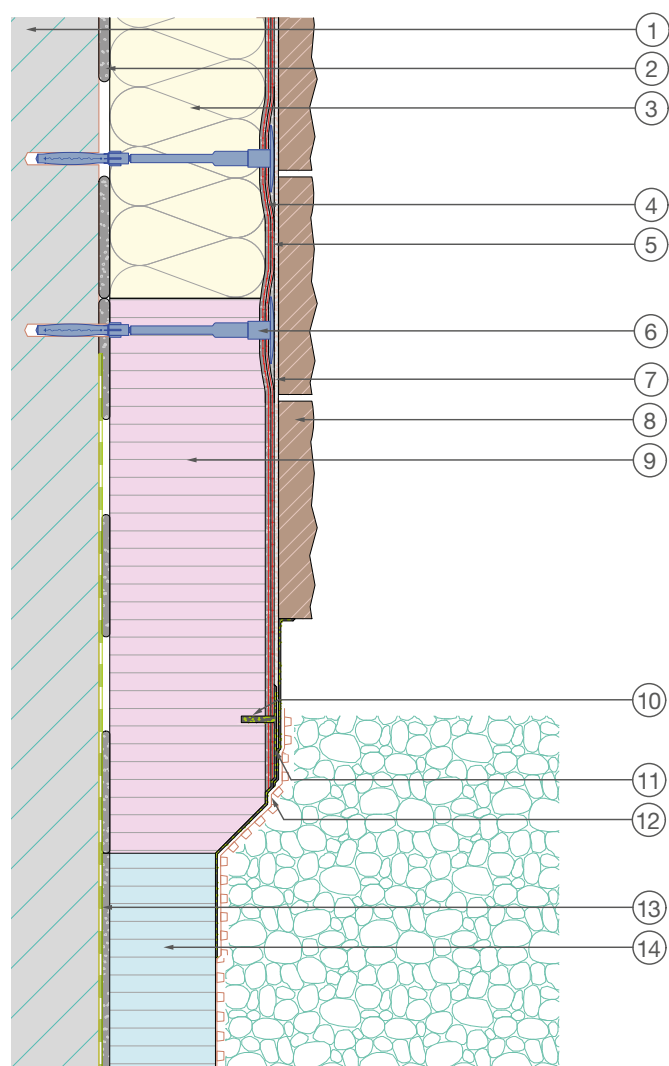
Detalj Omjer 1:2
