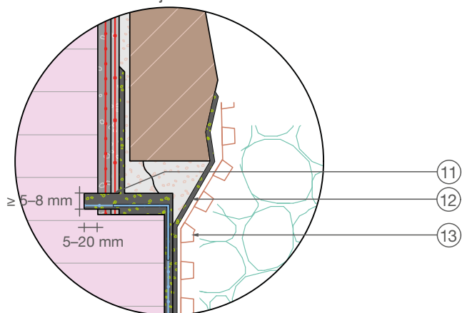
Detalj Omjer 1:2
