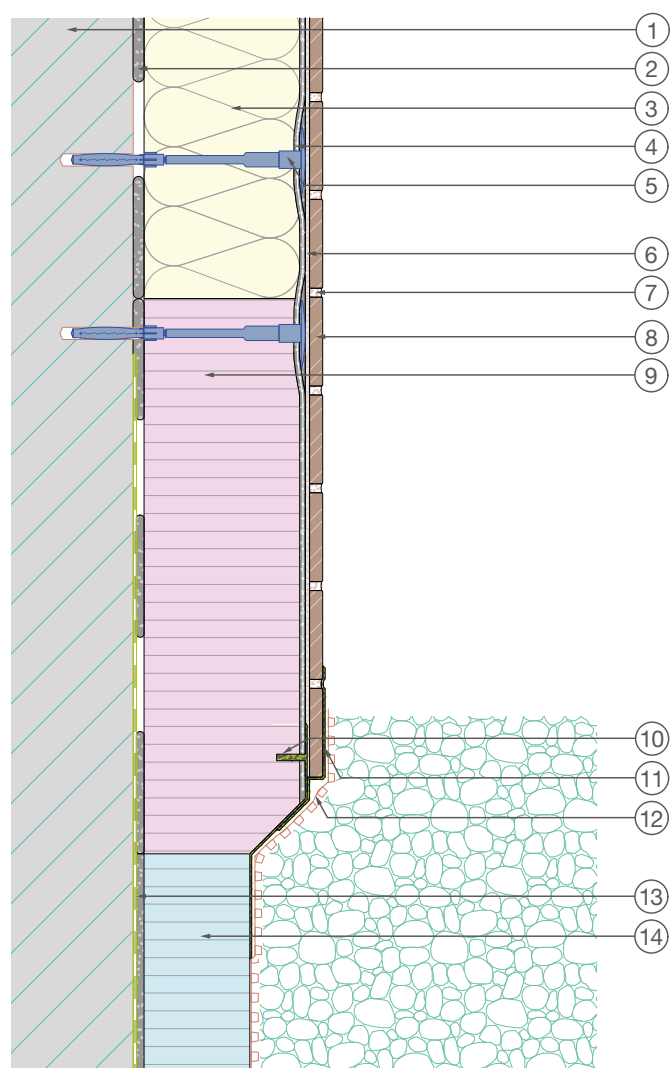
Detalj Omjer 1:2
