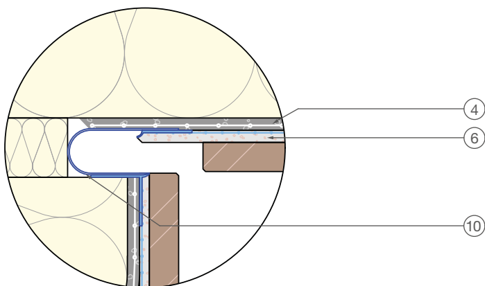
Detalj Omjer 1:2
